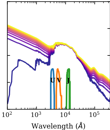
Quiescent
